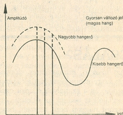
2. ábra Mintavétel különböző frekvenciájú és nagyságú analóg jelekből
