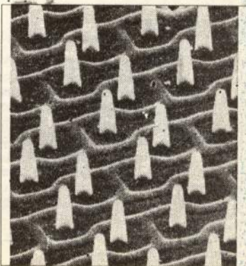
Egy 4 Mbit-es tároló elektronmikroszkóp alatt
