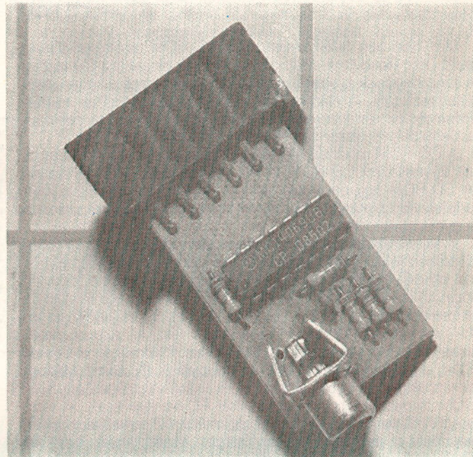
2. kép: Ez a kis adapter illeszti a CD lejátszót a C64-hoz. Az átviteli sebesség több mint 2,5-szer jobb, mint egy Turbo Tape, vagy akár egy 1541 esetén.
