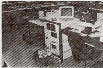
1. kép: A lemez mérőpad: a Media Logic ML2000
