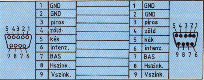
6. kép: Egy RGB digitális monitor csatlakoztatása kilencpólusú csatlakozóval. (A C128-as 80 karakteres módjához)
