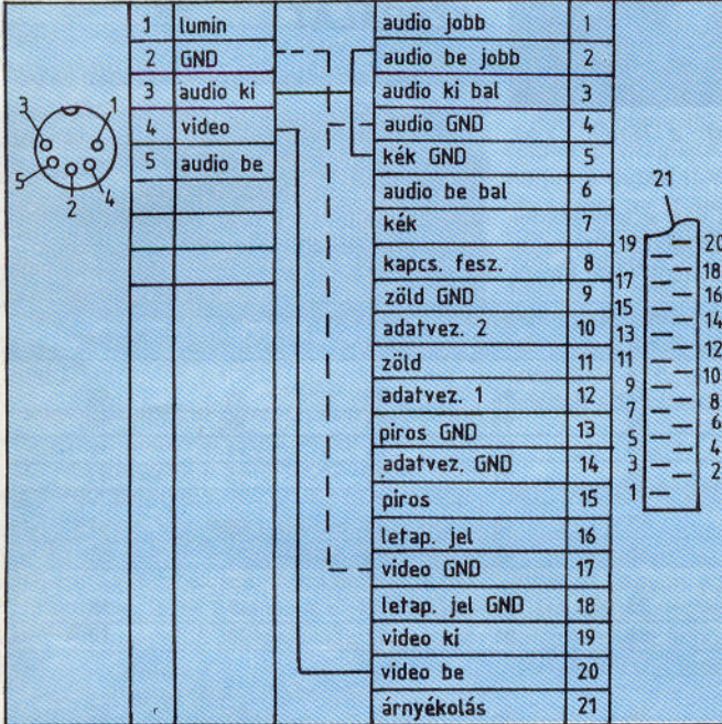
5. kép: Egy C64-es vagy egy C128-as csatlakoztatása egy tv vagy monitor Scart csatlakozójához (FBAS jel).
