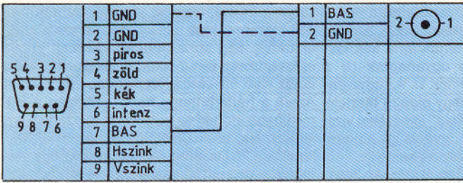
3. kép: Egy monokróm monitor csatlakoztatása a C128-as 80 karakteres képernyőjéhez.
