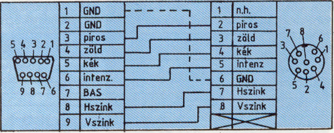
7. kép: Egy RGB digitális monitor csatlakoztatása nyolcpólusú DIN csatlakozáson keresztül a C128-hoz (80 karakteres üzemód.)
